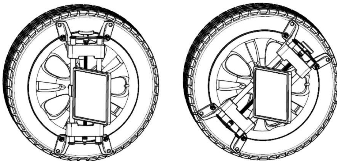
Рисунок 5.13 - Закрепление адаптера на колесе
